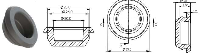
P571 - Tampão Universal
