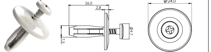
P624 - Grampo Universal
