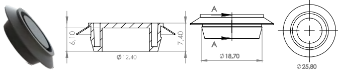
P555 - Tampão Universal
