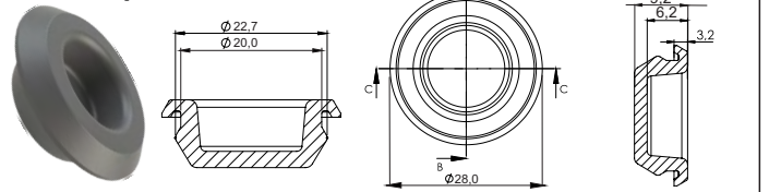
P573 - Grampo Universal
