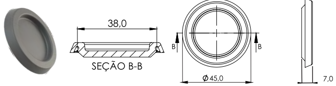
P565 - Tampão Universal
