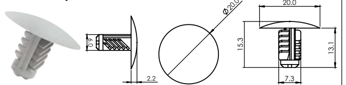
P622 - Grampo Universal
