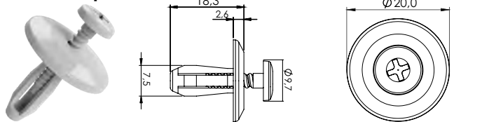
P625 - Grampo Universal
