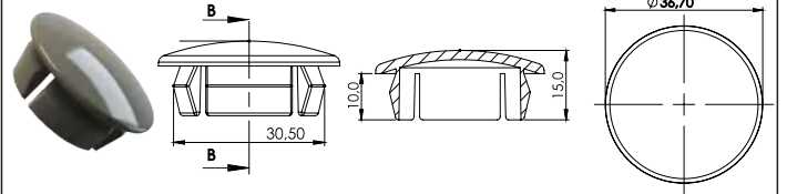
P564 - Tampão Universal
