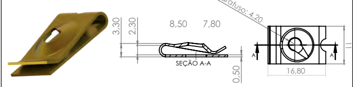
T33 - Presilha Metálica Universal
