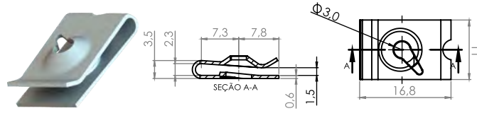
T29 - Porca Rápida Universal
