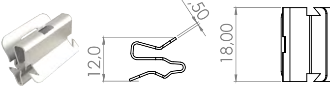
T36 - Presilha Metálica Universal
