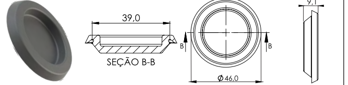
P566 - Tampão Universal
