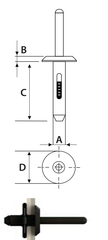
Detalhe da Peça Aplicada
