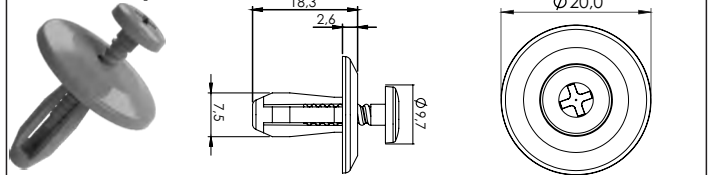
P570 - Tampão Universal
