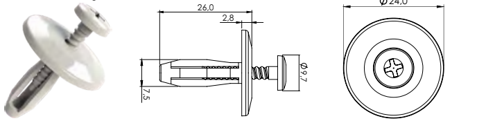
P569 - Tampão Universal
