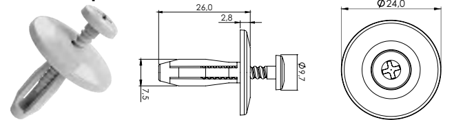
P623 - Grampo Universal
